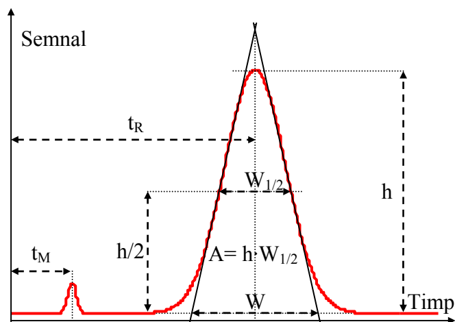
Fig. 4.8. Elementele unei cromatograme
