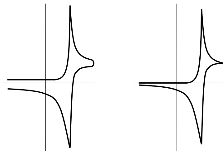
Fig. 7.10. Influența impurităților asupra CV: (a) cu, (b) fără impurități
