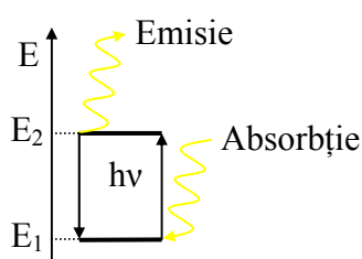
Fig. 6.1. Emisia și absorbția radiației în substanță
