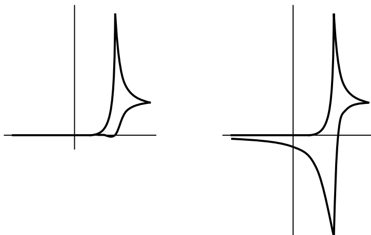
Fig. 7.9(a și b). Voltamograme ciclice la diferite viteze de variație a potențialului pentru (7.2) și (7.3)
