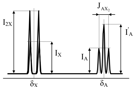
Fig. 5.6. Intensitatea diferită a cuplajelor spin-spin în spectrele AX și AX 2
