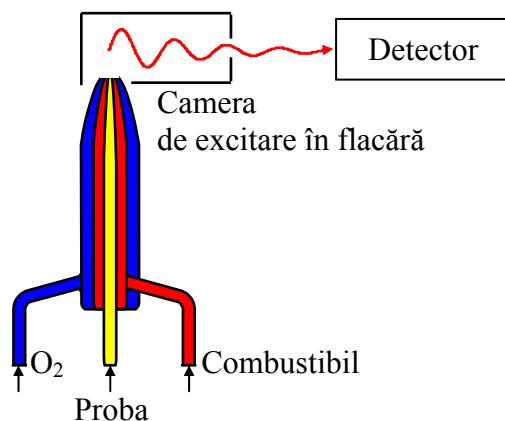
Fig. 6.12. Schema unui flamfotometru
