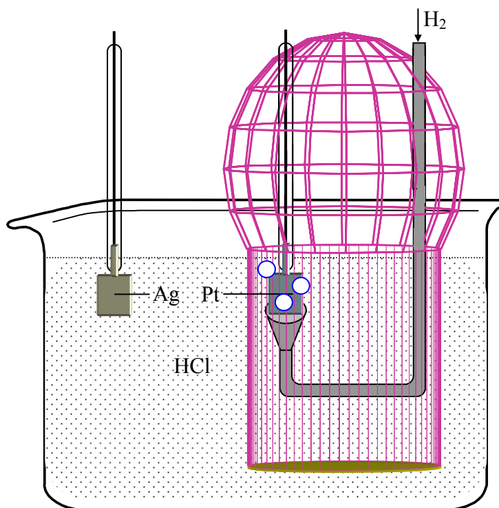
Fig. 8.4. Celulă galvanică cu electrolit comun
