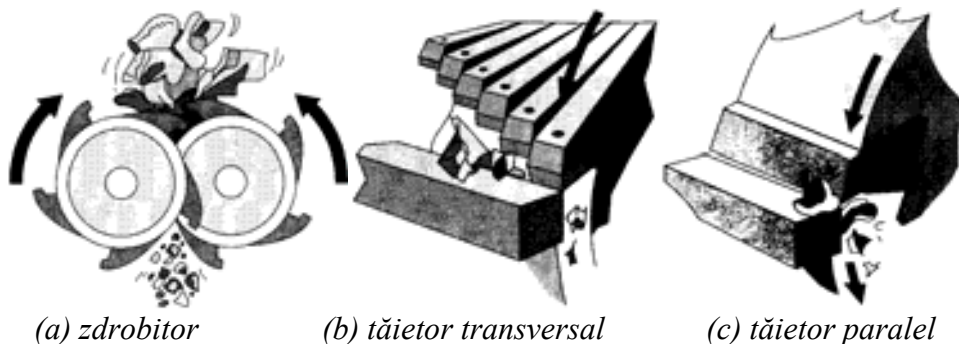
Fig. 2.2. Dispozitive de reducere a probei
