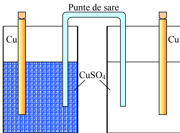
Fig. 8.6. Pilă de concentrație de electrolit
