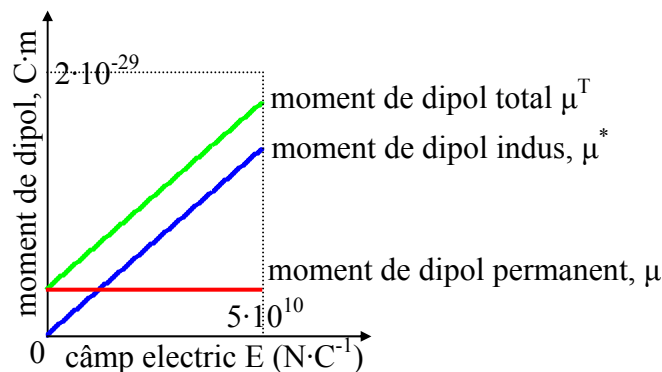
Fig. 6.6. Contribuțiile momentului de dipol indus și permanent la momentul de dipol electric total pentru \text{HCl} , 1 D = 3.336 \cdot 10^{-30} \text{ C}\cdot\text{m}
