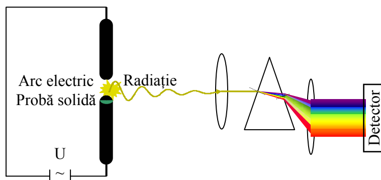
Fig. 6.13. Principiul metodei de excitație în arc electric
