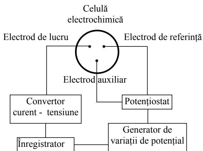
Fig. 7.6. Schema circuitului exterior în voltametrie ciclică
