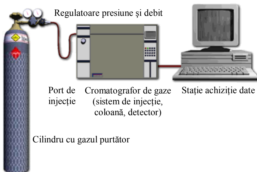
Fig. 4.4. Aparatura pentru cromatografia de gaze
