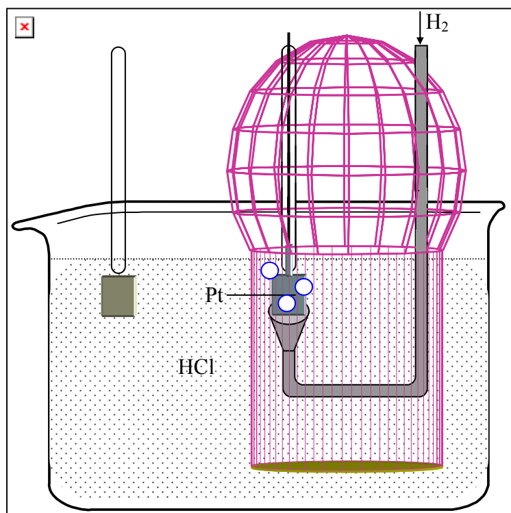
Fig. 8.4. Celulă galvanică cu electrolit comun
