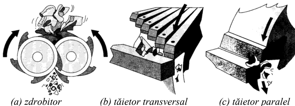
Fig. 2.2. Dispozitive de reducere a probei
