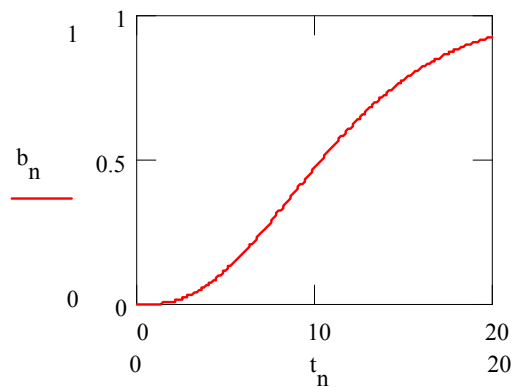
Fig. 7.11. Dependența concentrației de produs [B]=b_n în timp ( t_n )
