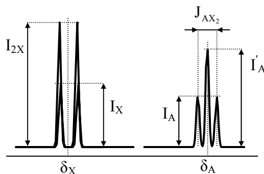
Fig. 5.6. Intensitatea diferită a cuplajelor spin-spin în spectrele AX și AX_2
