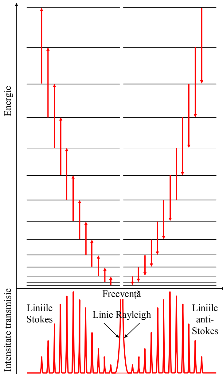
Fig. 6.7. Nivele energetice de rotație, tranziții permise de \Delta J = \pm 2 și spectru de rotație Raman tipic
