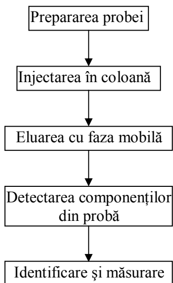
Fig. 4.5. Faze în HPLC
