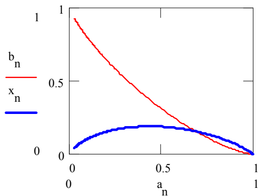
Fig. 7.12. Dependența concentrației de produs ( b_n ) și intermediar ( x_n ) în funcție de cantitatea de reactant ( a_n )
