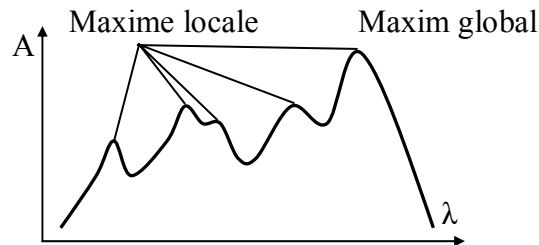
Fig. 6.3. Dependența absorbției de lungimea de undă a radiației
