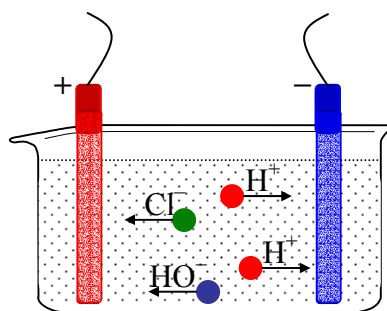
Fig. 8.8. Electroliza soluției apoase de HCl
