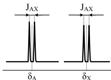
Fig. 5.5. Efectul cuplajului spin-spin asupra unui spectru AX
