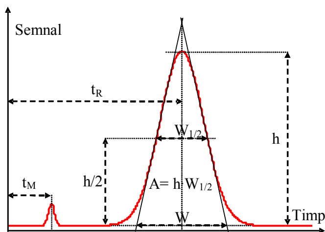
Fig. 4.8. Elementele unei cromatograme
