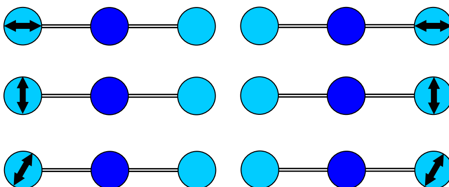
Fig. 6.11. Vibrațiile atomilor de oxigen în jurul pozițiilor de echilibru în molecula de CO 2 după cele 3 axe (Ox, Oy, Oz) ale sistemelor de referință locale fixate pe atomi
