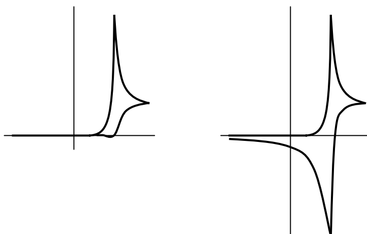
Fig. 7.13(a și b). Voltamograme ciclice la diferite viteze de variație a potențialului pentru (7.2) și (7.3)
