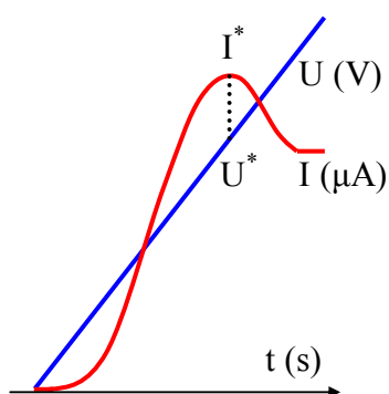
Fig. 7.3. Diagramele tensiune-timp și curent-timp într-un experiment de voltametrie liniară
