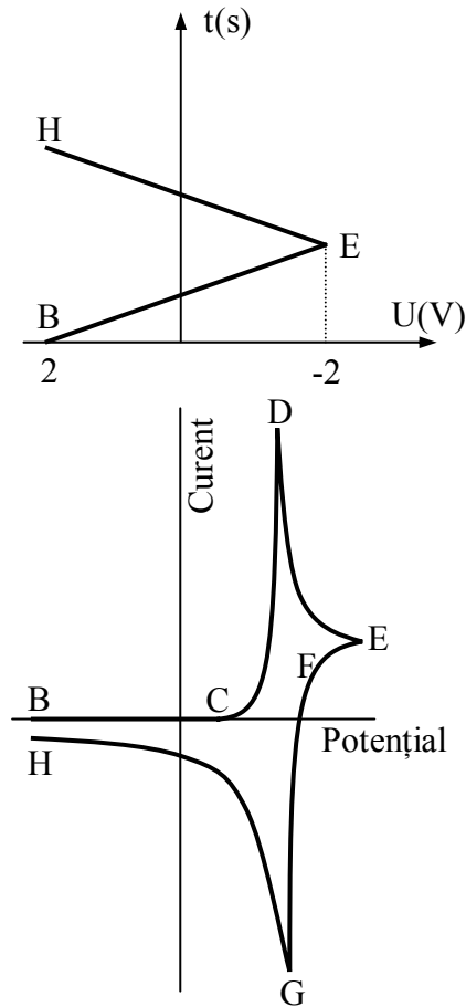
Fig. 7.7. Forma unei voltamograme ciclice
