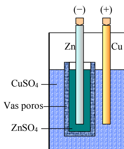
Fig. 8.5. O variantă a pilei Daniel
