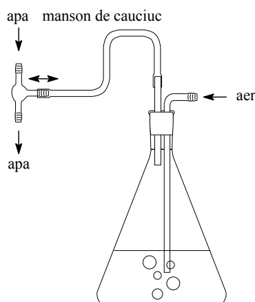
Fig. 2.1. Instalație pentru probe de aer
