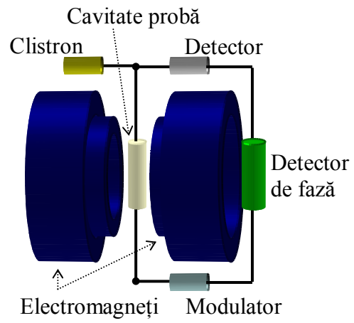
Fig. 5.12. Schema bloc a unui spectrometru RES
