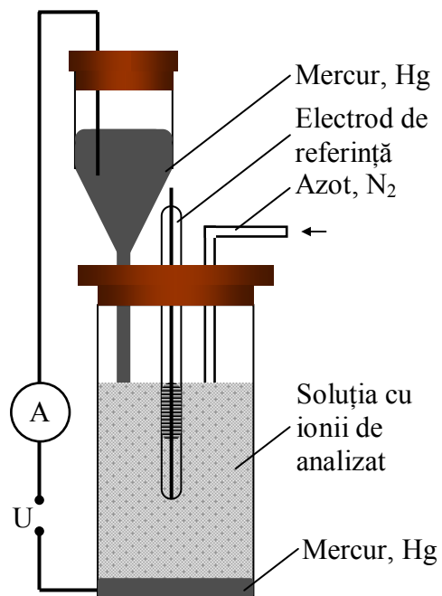
Fig. 7.1. Principiul polarografiei
