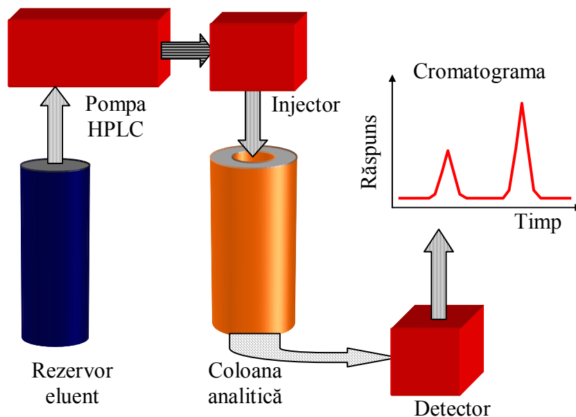
Fig. 4.6. Schema Bloc a HPLC
