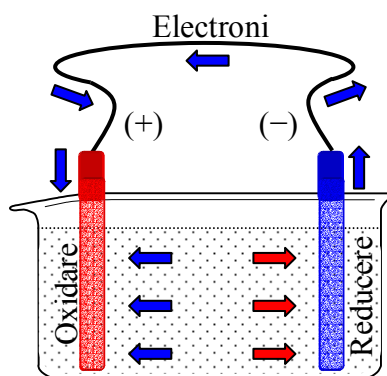
Fig. 8.2. Circulația purtătorilor de sarcină într-o celulă electrochimică și în circuitul exterior acesteia
