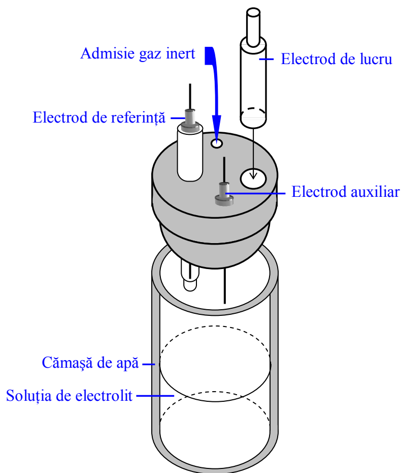
Fig. 7.5. Schema unei instalații de voltametrie ciclică
