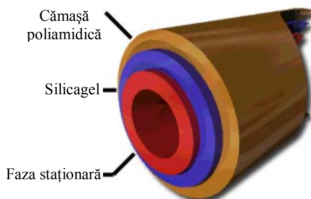
Fig. 4.2. Secțiune prin coloana de separare
