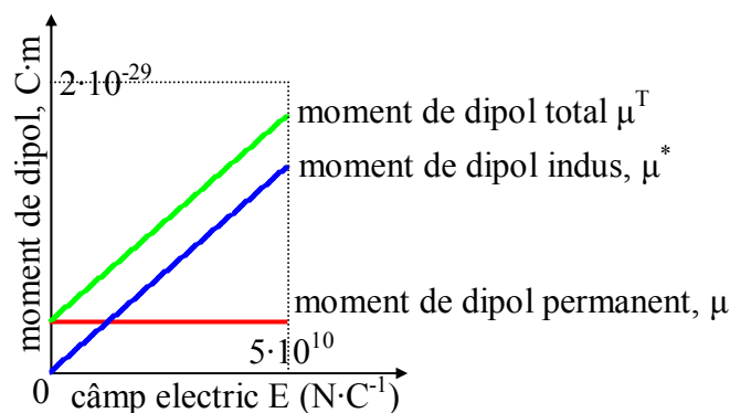
Fig. 6.6. Contribuțiile momentului de dipol indus și permanent la momentul de dipol electric total pentru \text{HCl} , 1 D = 3.336 \cdot 10^{-30} \text{ C} \cdot \text{m}
