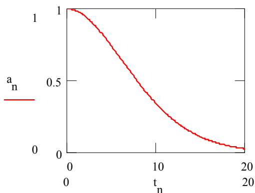
Fig. 7.9. Dependența concentrației de reactant [A] = a_n în timp ( t_n )
