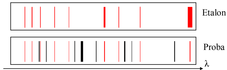
Fig. 6.14. Compararea spectrului probei cu spectrul etalonului
