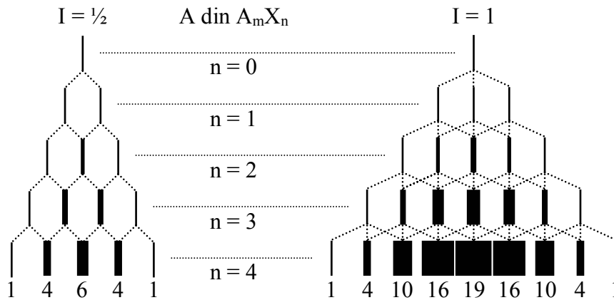
Fig. 5.7. Cuplaje spin-spin scindări și suprapuneri pentru semnalul lui A din A_mX_n
