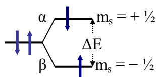
Fig. 5.11. Nivelele de spin electronic în câmp magnetic
