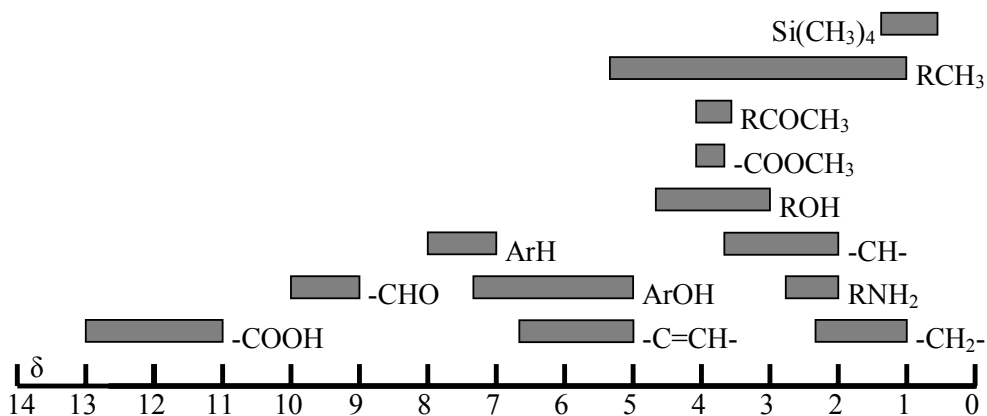
Fig. 5.2. Domeniul de deplasări chimice \delta ale ^1\text{H} în diferite grupări funcționale
