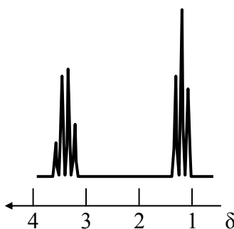
Fig. 5.10. Interpretarea unui spectru ^1\text{H} -RMN
