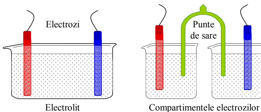
Fig. 8.1. Celule electrochimice
